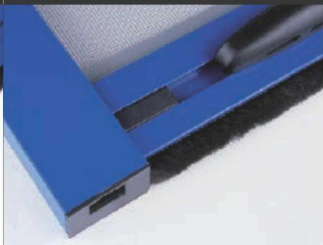
Equerre invisible pour fixation de la lame finale
